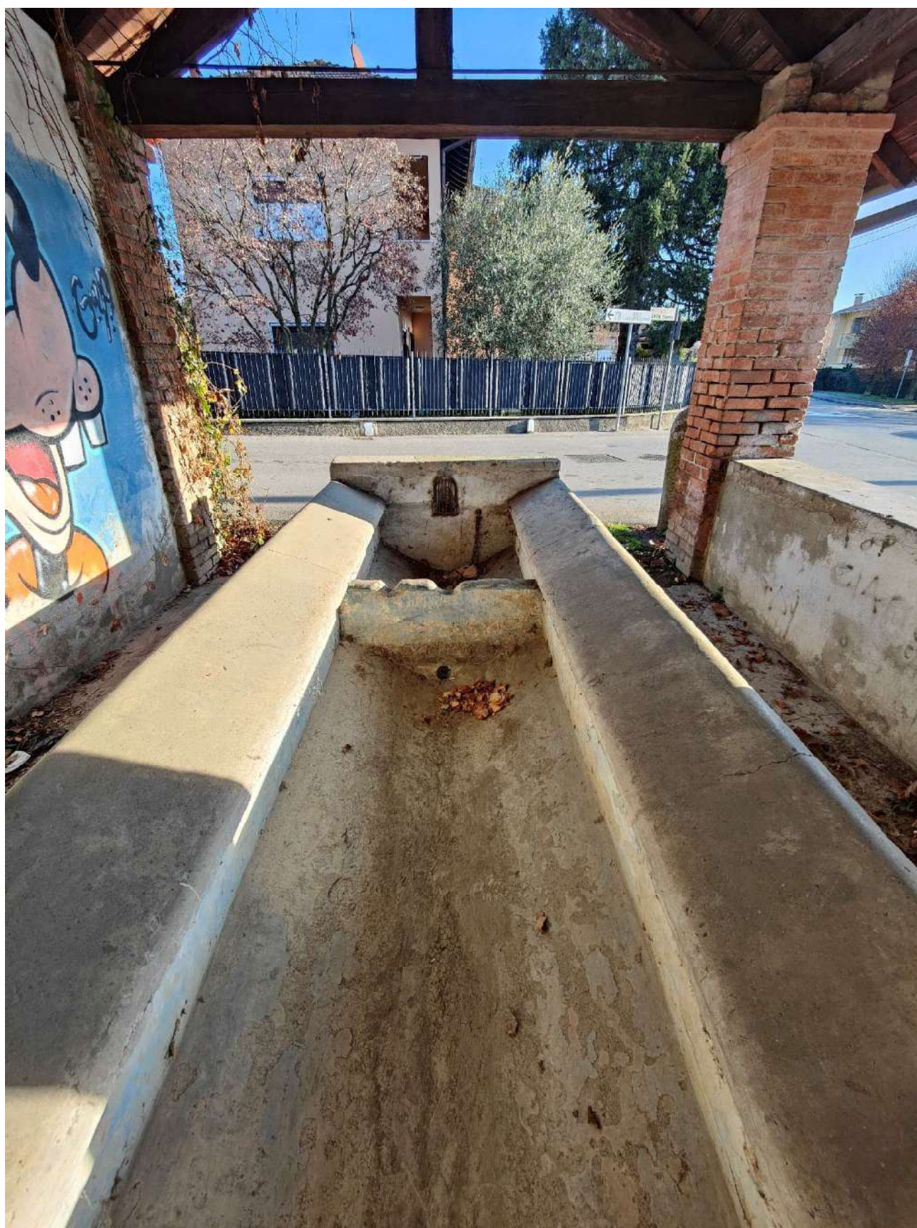
Elemento di separazione tra le vasche e scarico di troppo pieno
